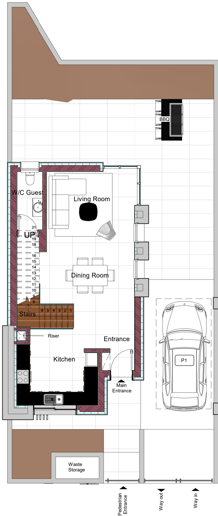
Level 0 FFL (P) 1 : 100
