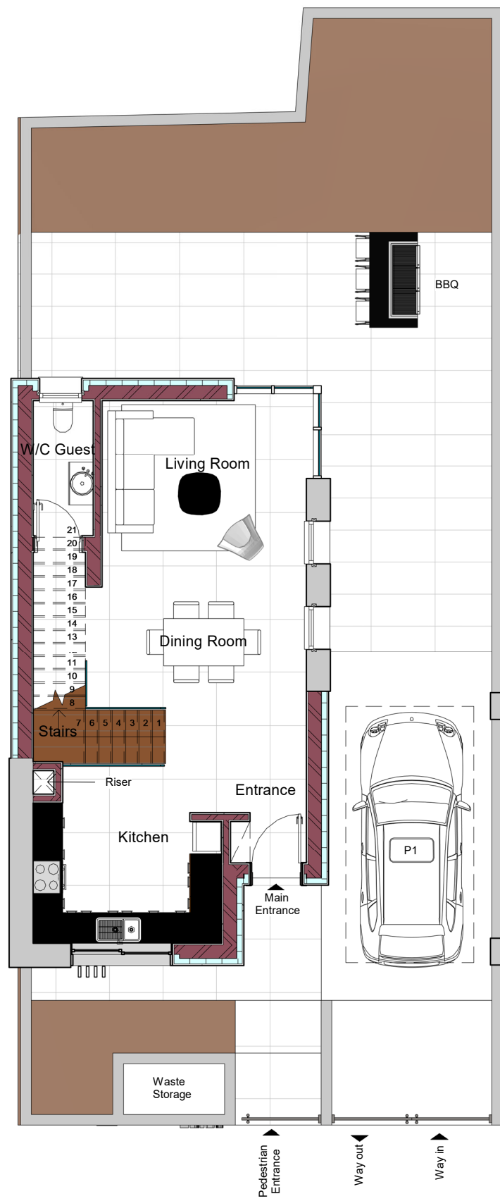
Level 0 FFL (P) 1 : 100
