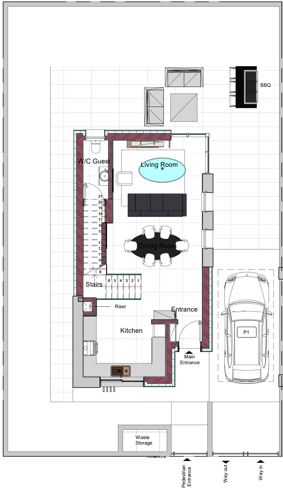
Level 0 FFL (P) 1 : 100
